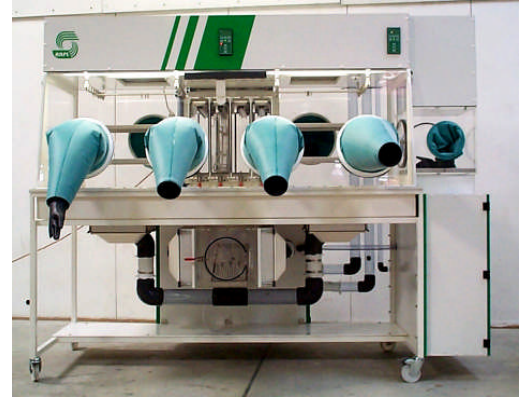
ISOLATEUR ISOPLEX OSSATURE RIGIDE
